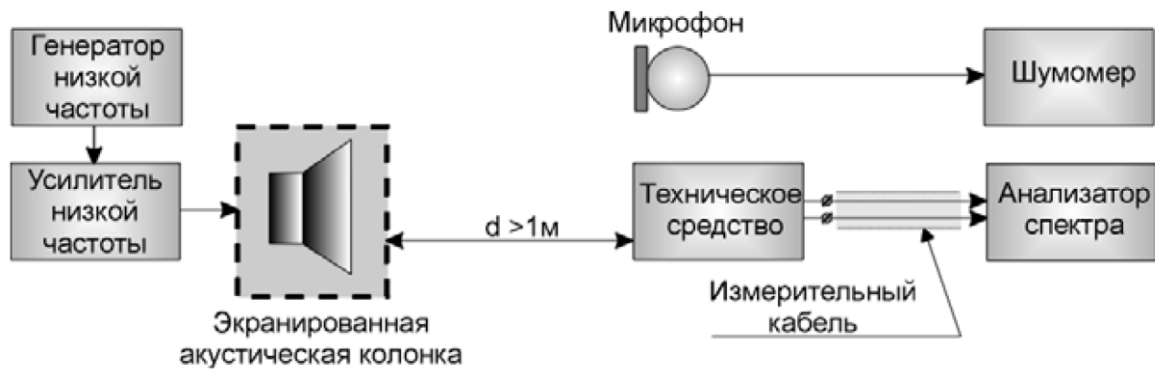
Рис. 3.3. Блок-схема измерительного стенда
